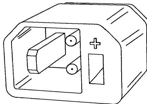
图 1 铅酸蓄电池充电器输出插头形式
